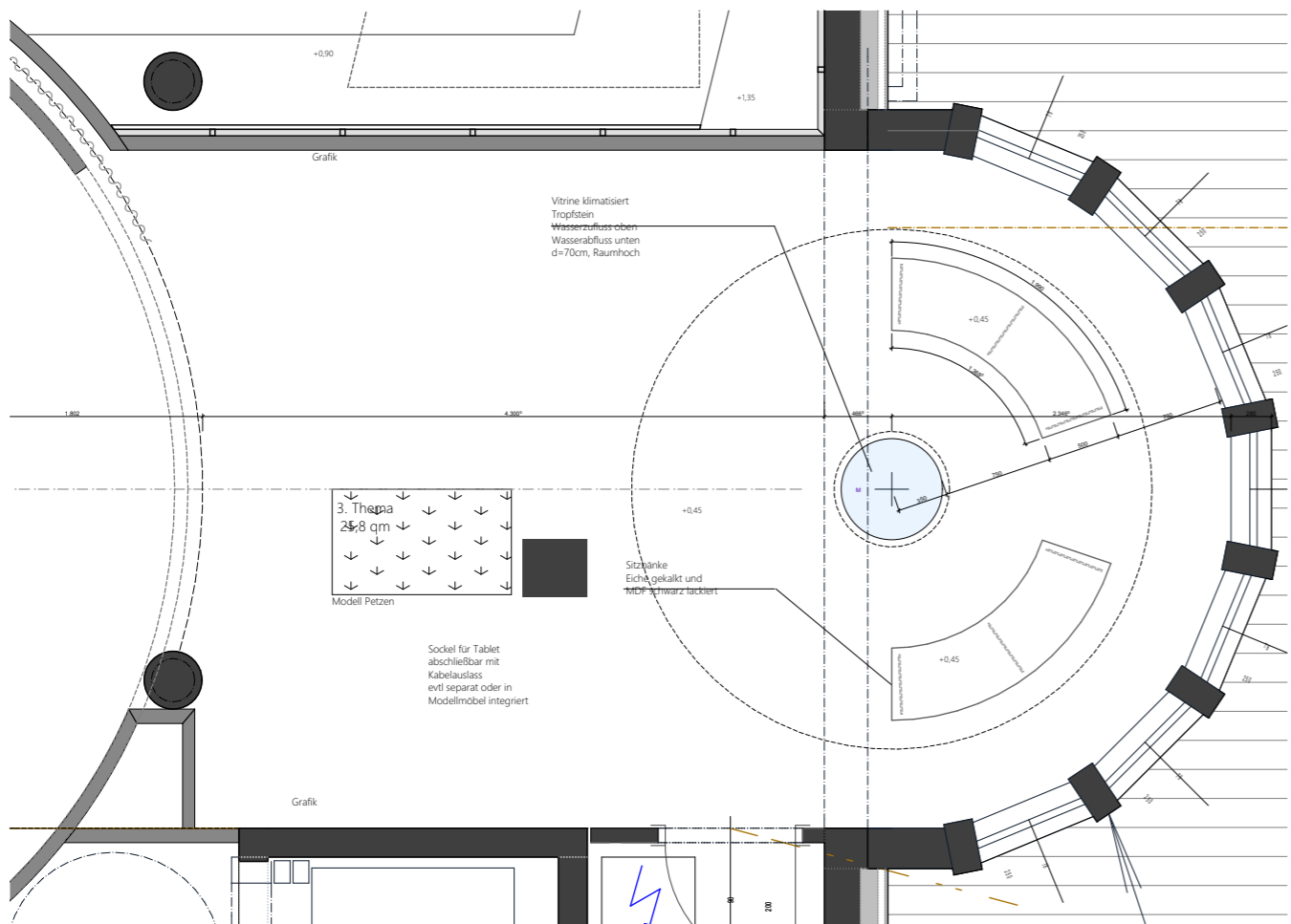
Grundriss
